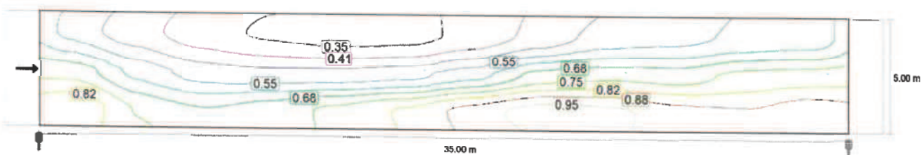
Observator 1: Densitatea luminii la instalația nouă [ \text{cd}/\text{m}^2 ] (Linii Isolux)
