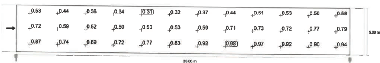
Observator 1: Densitatea luminii la instalația nouă [ \text{cd}/\text{m}^2 ] (Raster valoric)
